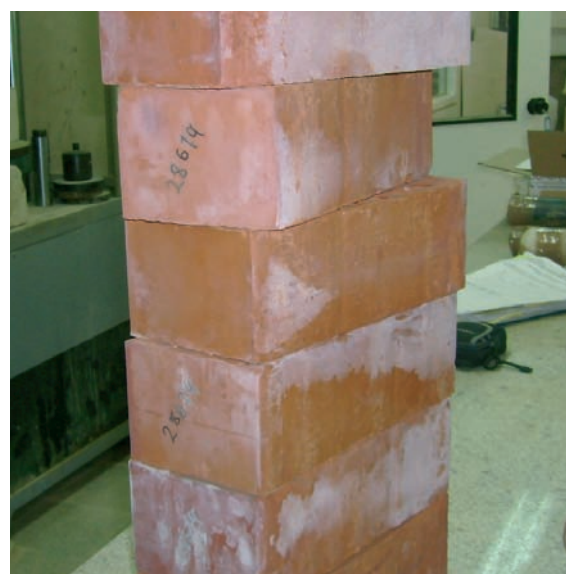
Assaig d'eflorescències.
