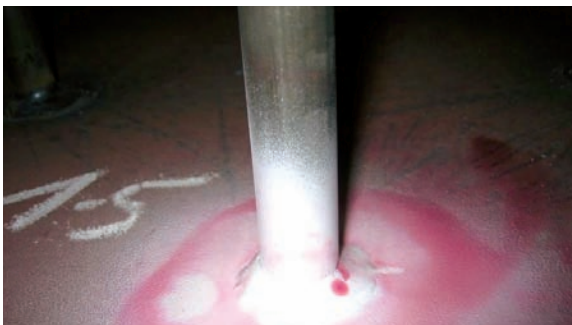
Inspecció no destructiva per a líquids penetrants.
